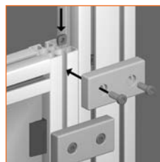
Anschlussplatten
